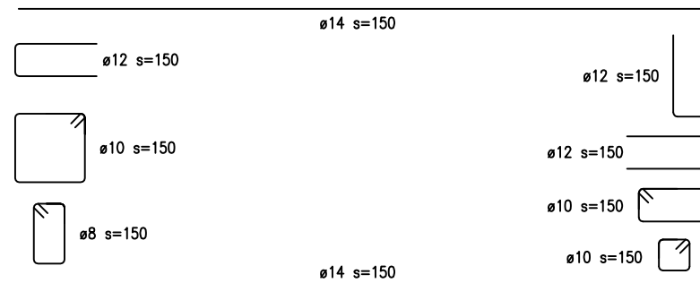
Querschnitt A-A / Coupe A-A W11 1/50
