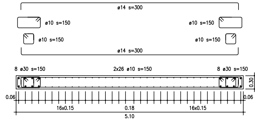
Querschnitt A-A / Coupe A-A W11 1/50
