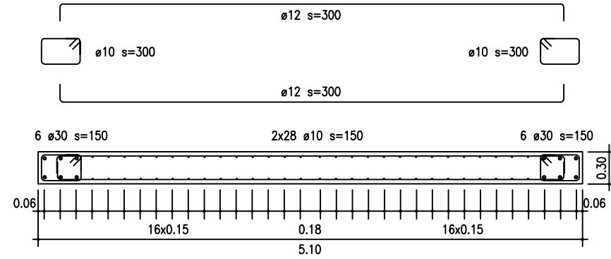
Querschnitt B-B / Coupe B-B W11 1/50
